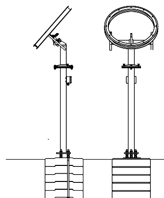
Nárys a bokorys stojanu pro snímač globálního záření se stínícím kruhem pro získání difúzního záření
